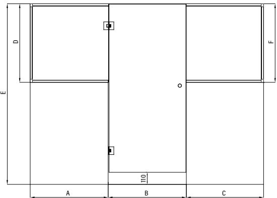
Vetro S49 Saunan lasiseinä vedin- ja saranapuolen siviikkunoilla
