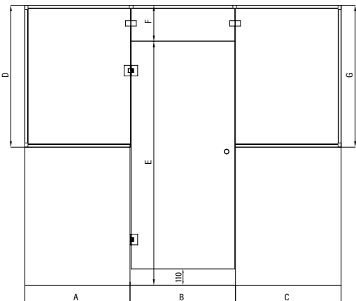
Vetro S51 Saunan lasiseinä vedin- ja saranapuolen siviikkunoilla ja yläikkunalla
