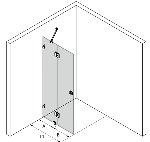
Vetro 514 Kääntyvä suihkuseinä kiinteällä osalla
